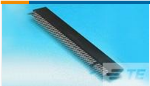
TE 系列/零件编号1-5530843-8 CONN SEC II 30 POS 100C /L
