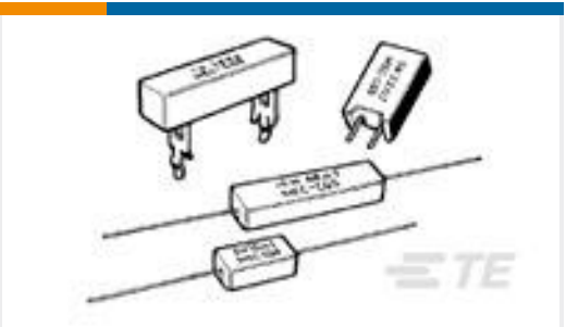
TE 系列/零件编号1-1623793-6 SQP5 33K 5% MTL FLM
