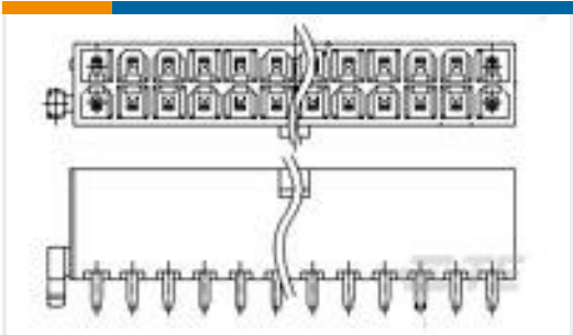
TE 系列/零件编号1-1775099-3 ATX PWR CONN 1 BDLK 24 POS
