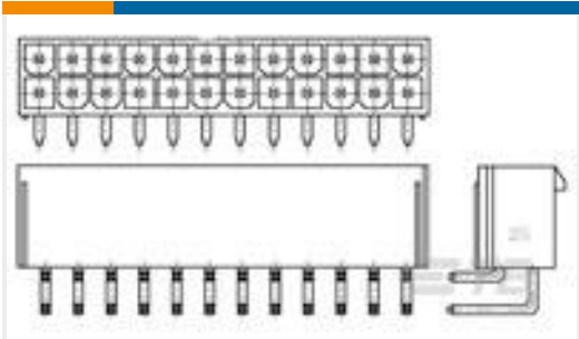
TE 系列/零件编号2-1586041-4 24P VAL-U-LOK R/A HDR V2
