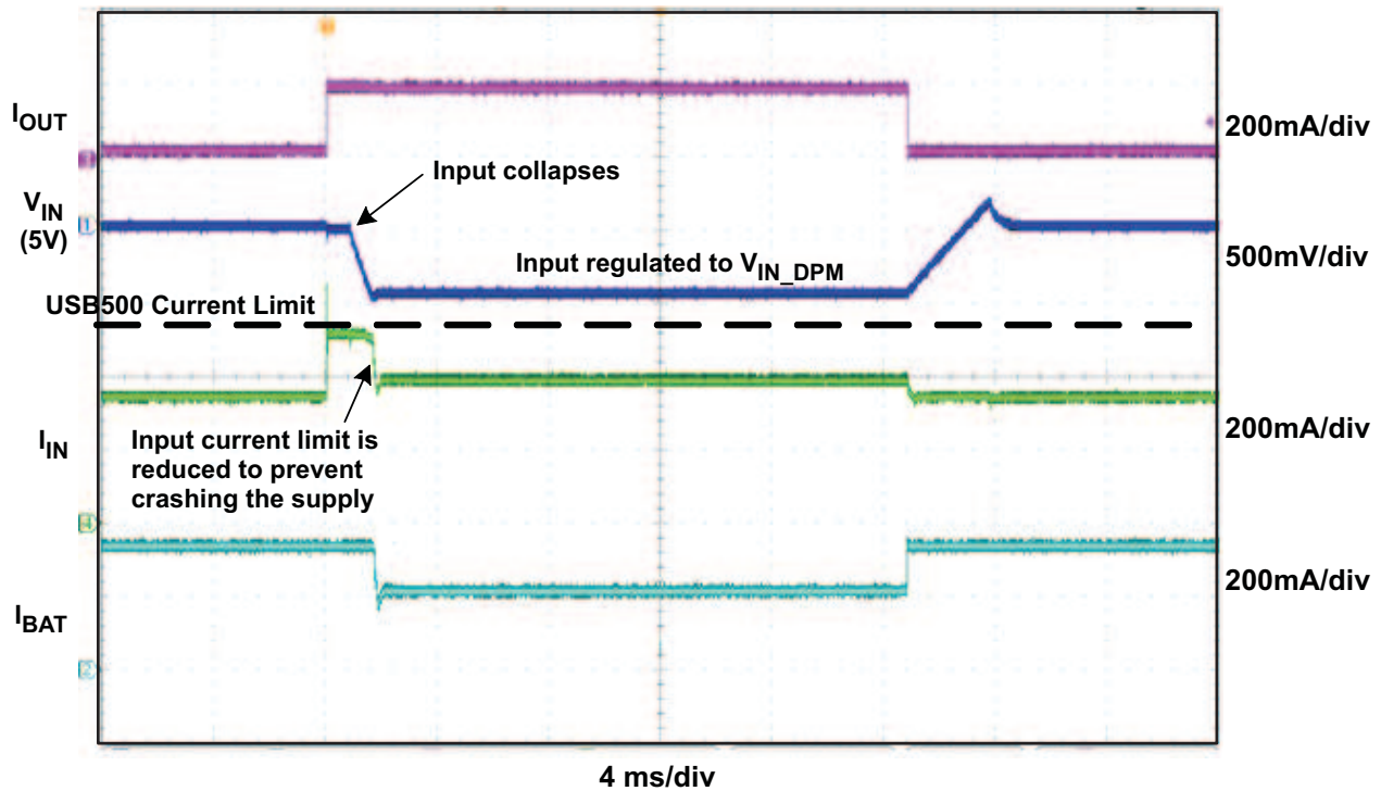
图 21. V_{IN-DPM} Waveform
