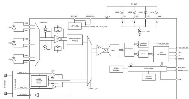
简化框图
