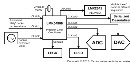
简化 LMK04906 方框图
