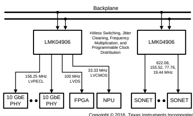
系统应用图
