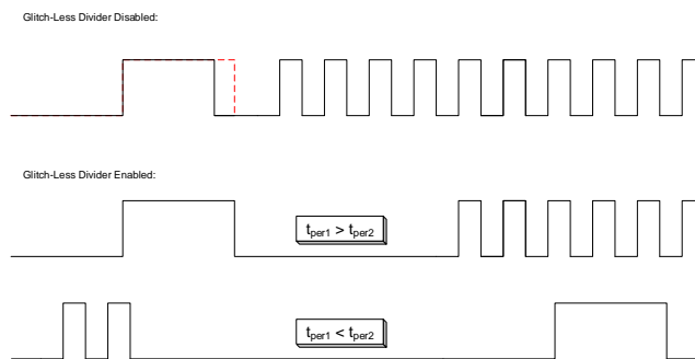
图 24. Glitch-Less Divider Update
