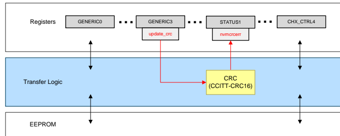
图 28. EEPROM CRC
