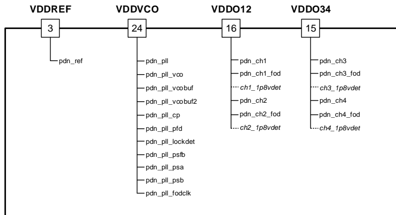
图 29. Power Management
