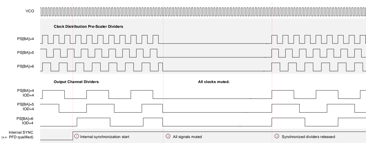
图 27. Divider Synchronization
