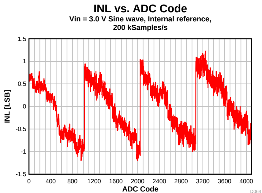
图 5-26. INL vs. ADC Code
