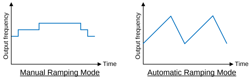
图 24. Ramping Modes
