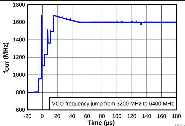
图 15. VCO Calibration Time
