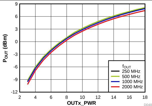
图 18. Configurable Output Power
