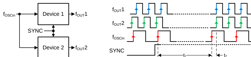
图 23. Phase Synchronization
