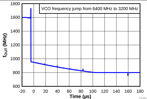
图 16. VCO Calibration Time
