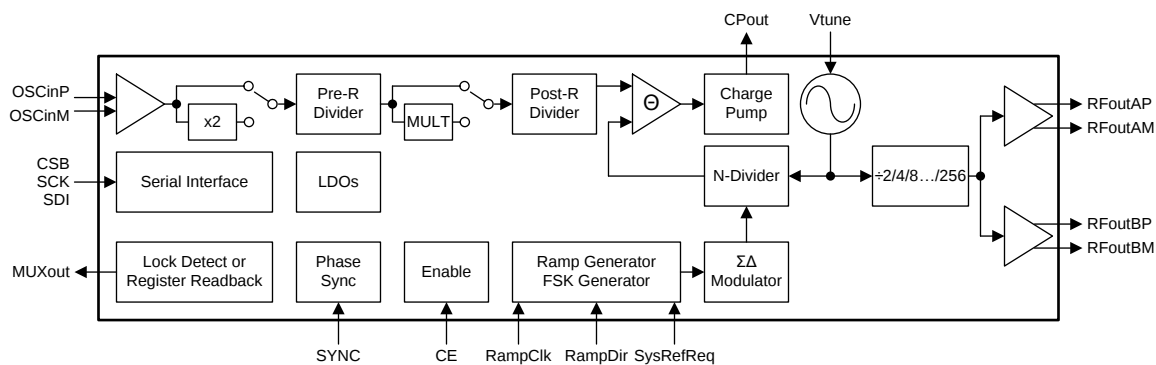
功能方框图
