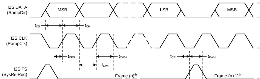
图 26. FSK I2S Timing Diagram
