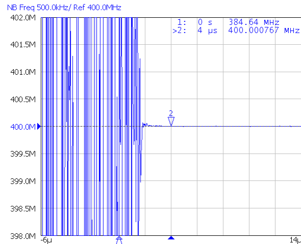
图 157. Buffer Power Up at 400-MHz Output
