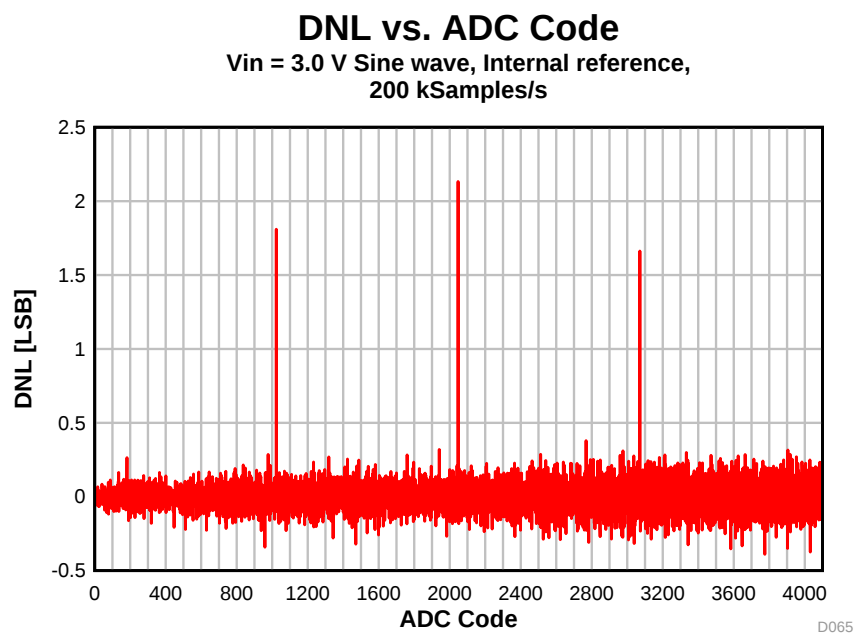
图 5-24. DNL vs. ADC Code
