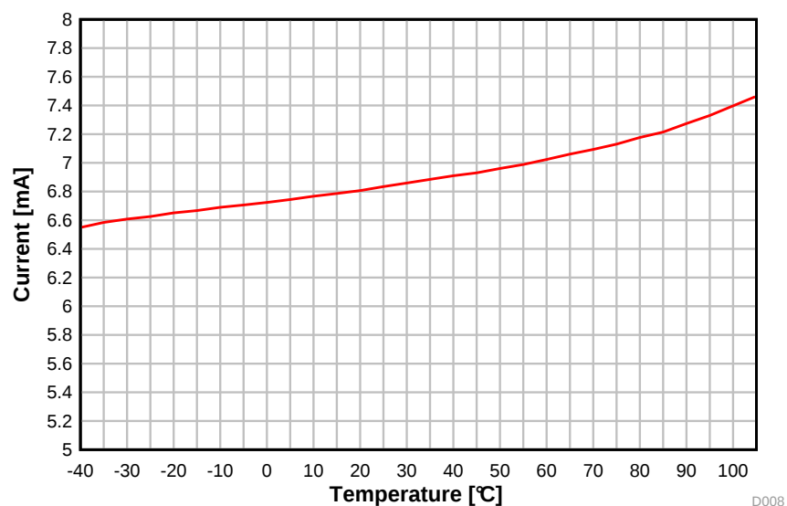
图 5-7. RX Current vs. Temperature (50 kbps, 868.3 MHz)
