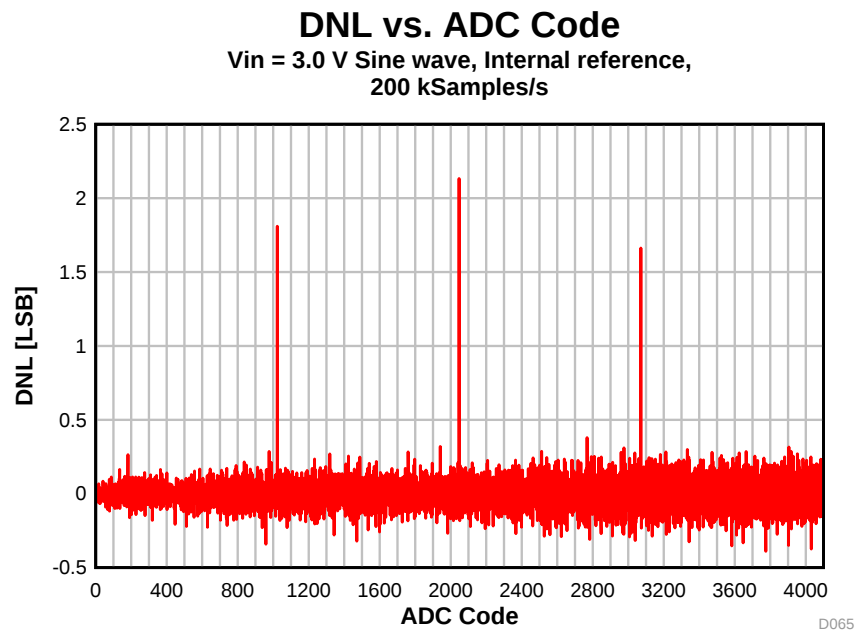
图 5-42. DNL vs. ADC Code
