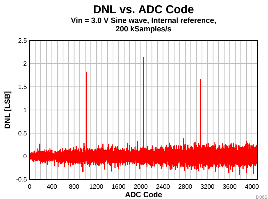
图 5-52. DNL vs. ADC Code
