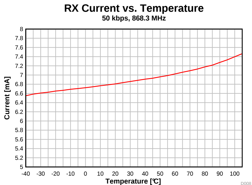
图 5-7. RX Current vs. Temperature (50 kbps, 868.3 MHz)
