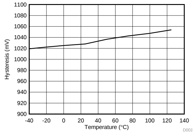
图 17. UVLO Hysteresis vs. Temperature
