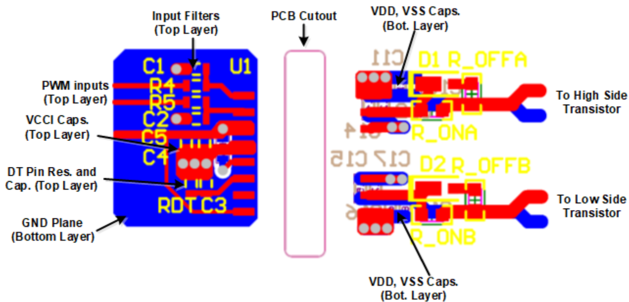
图 44. Layout Example
