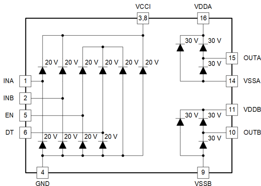
图 36. ESD Structure
