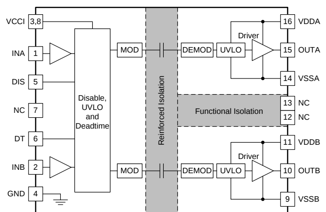
功能框图
