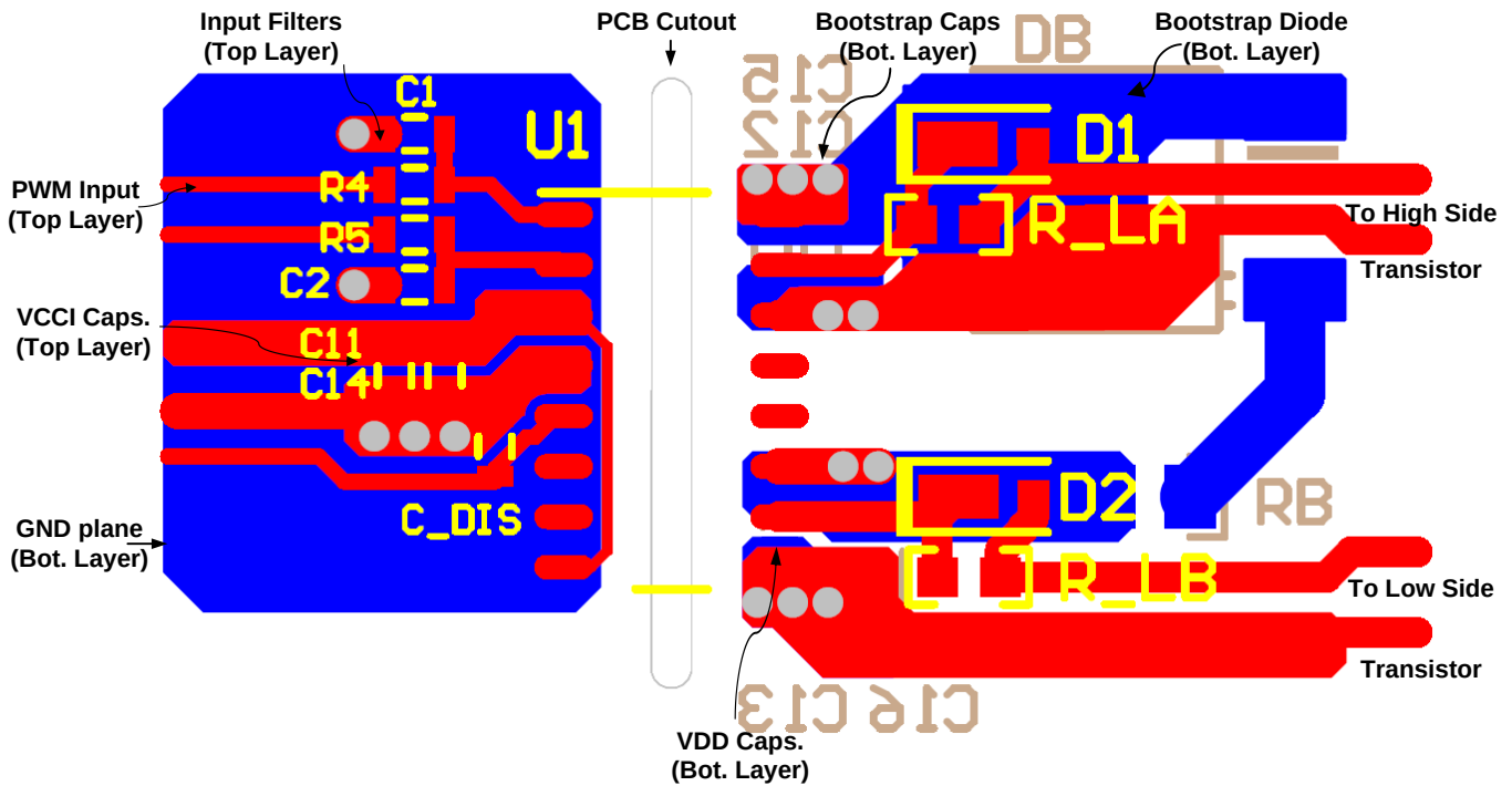
图 42. Layout Example
