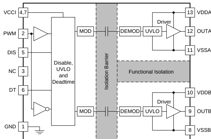
功能方框图
