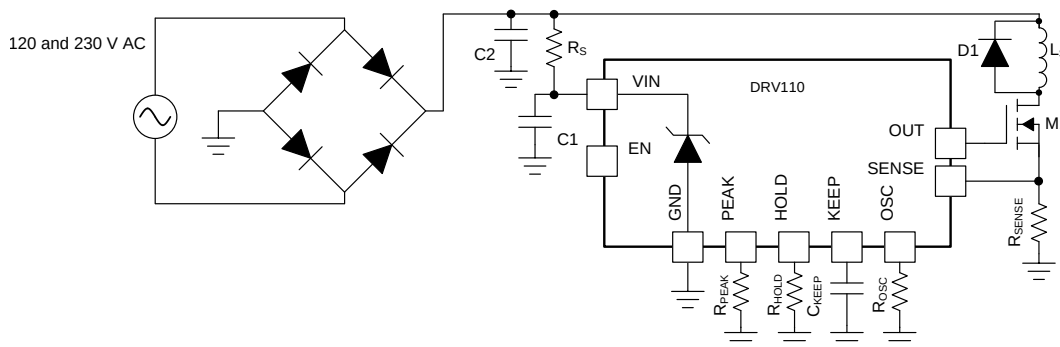
由电源线电压供电的 DRV110A-Q1
