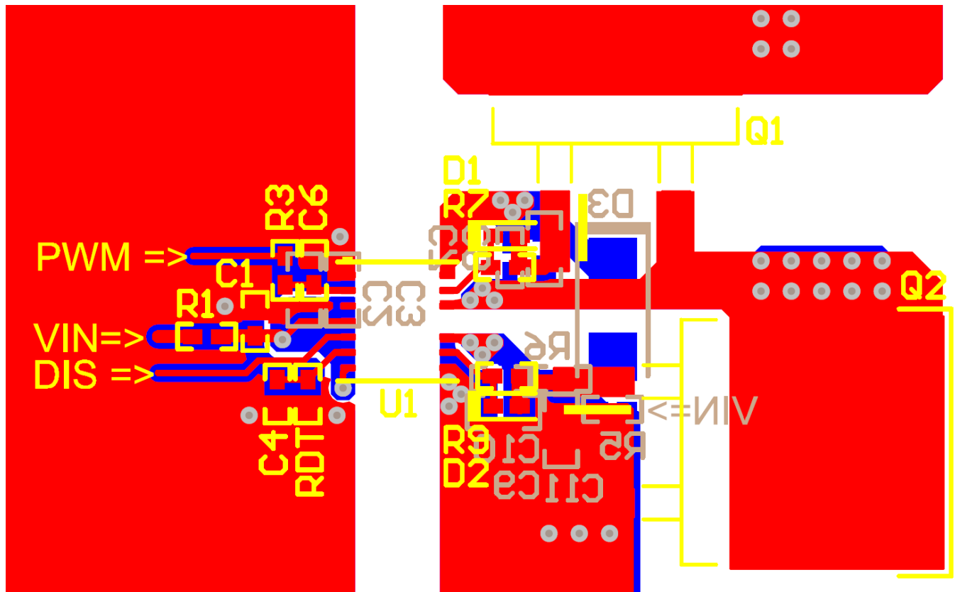
图 41. Layout Example
