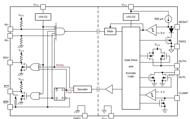
功能框图
