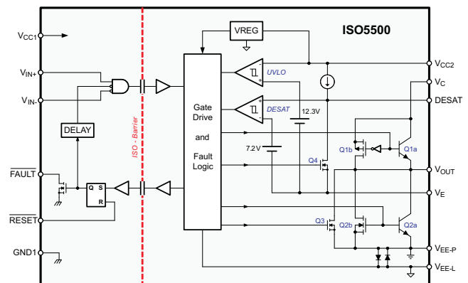
功能方框图
