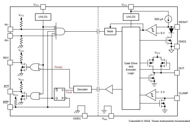
功能方框图
