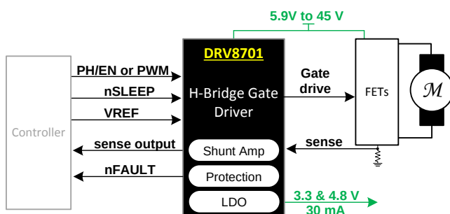
简化的系统框图
