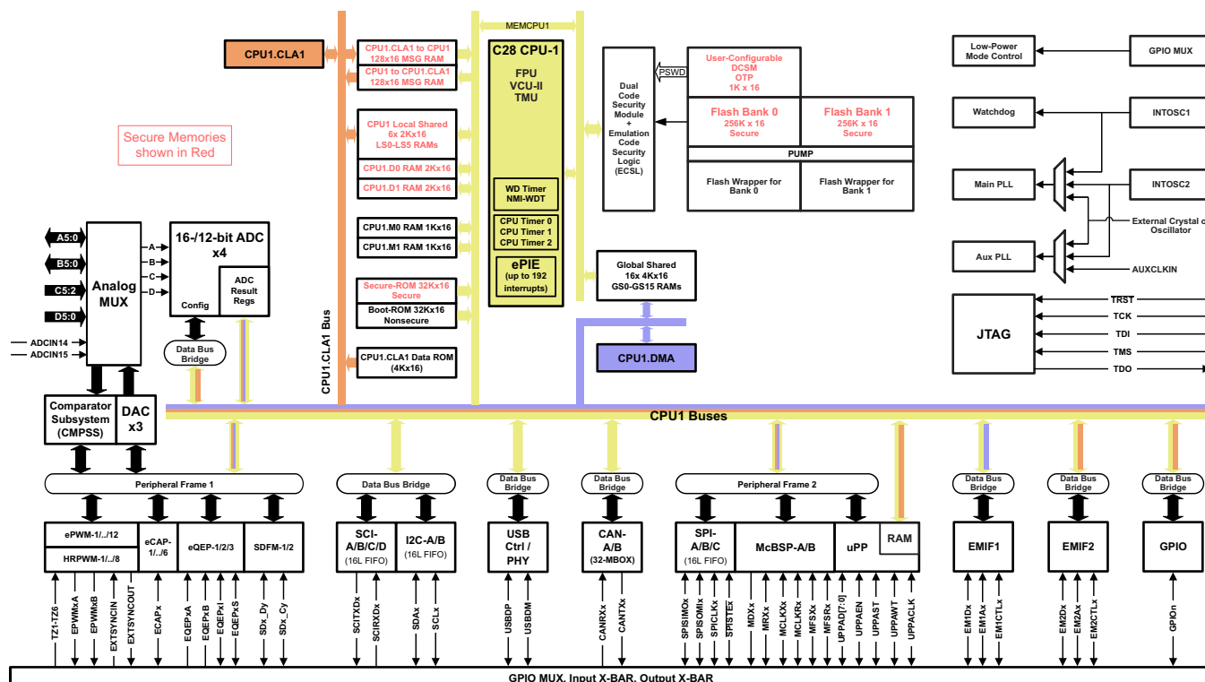
图 1-1. 功能方框图
