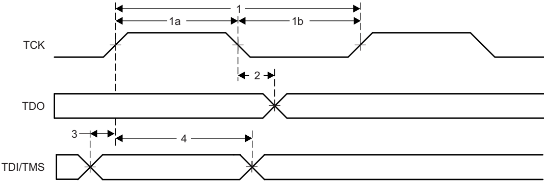
图 5-11. JTAG Timing
