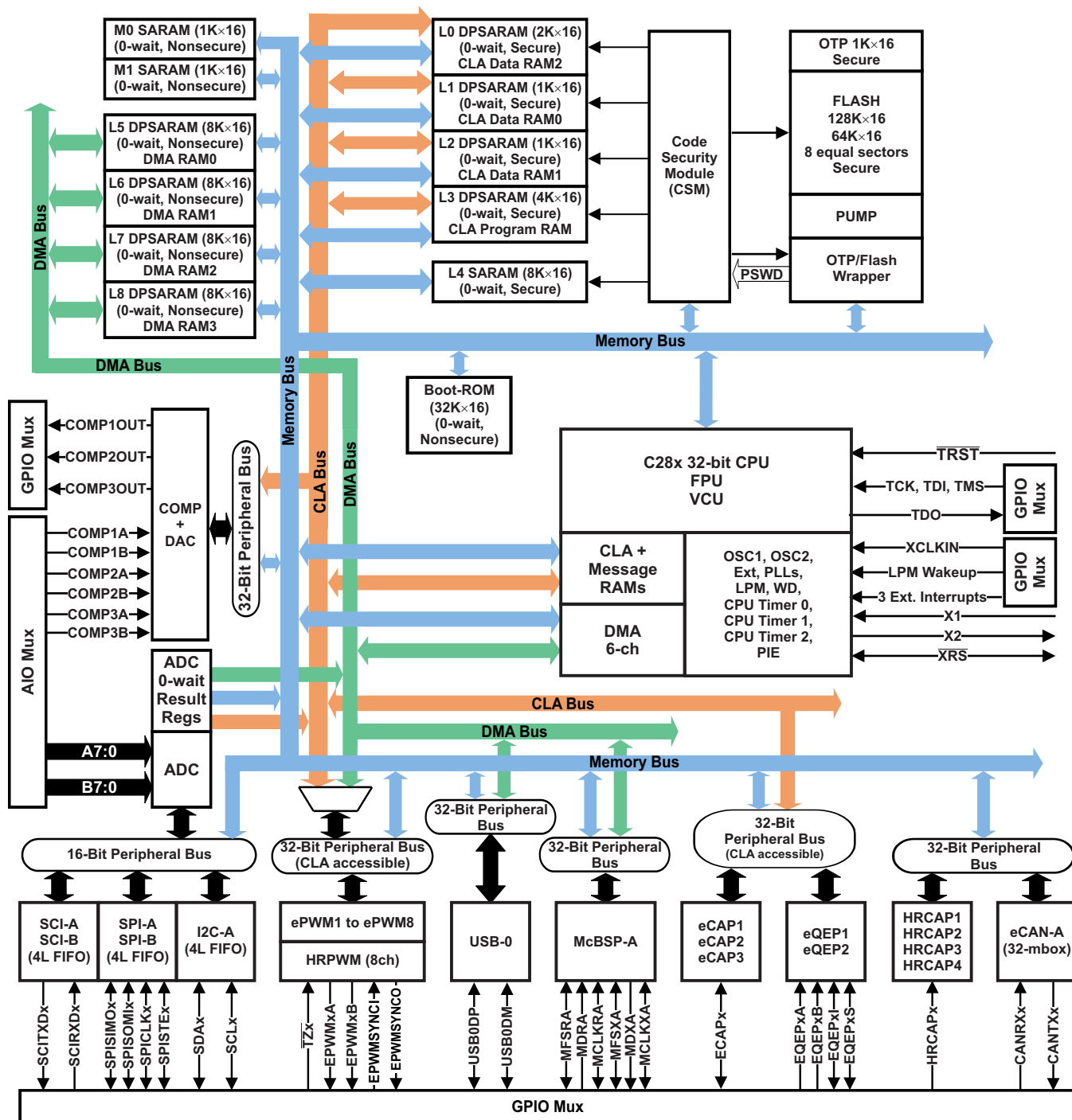
图 1-1. 功能方框图
