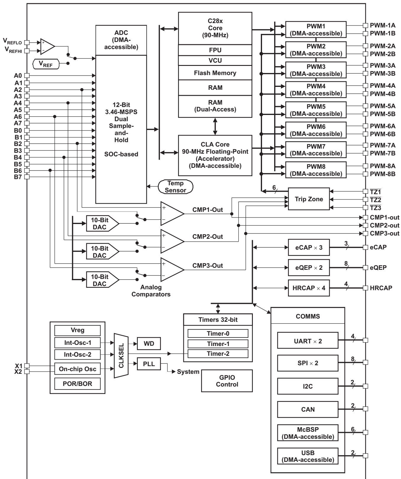
图 1-2. 外设块
