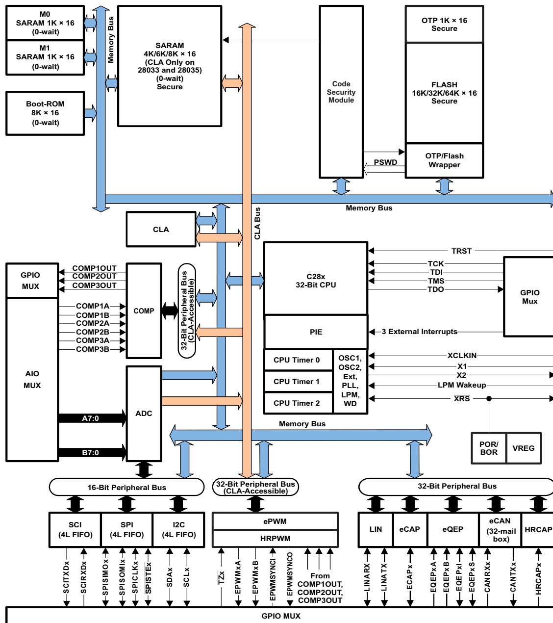
图 1-1. 功能方框图
