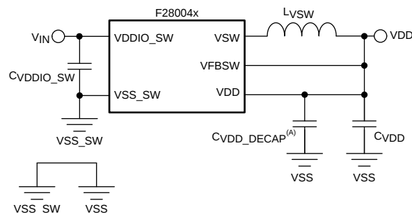
图 5-6. DC-DC Circuit Schematic
