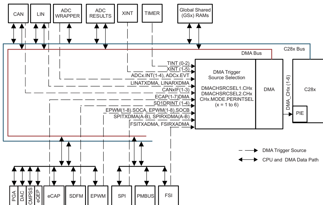
图 6-3. DMA Block Diagram
