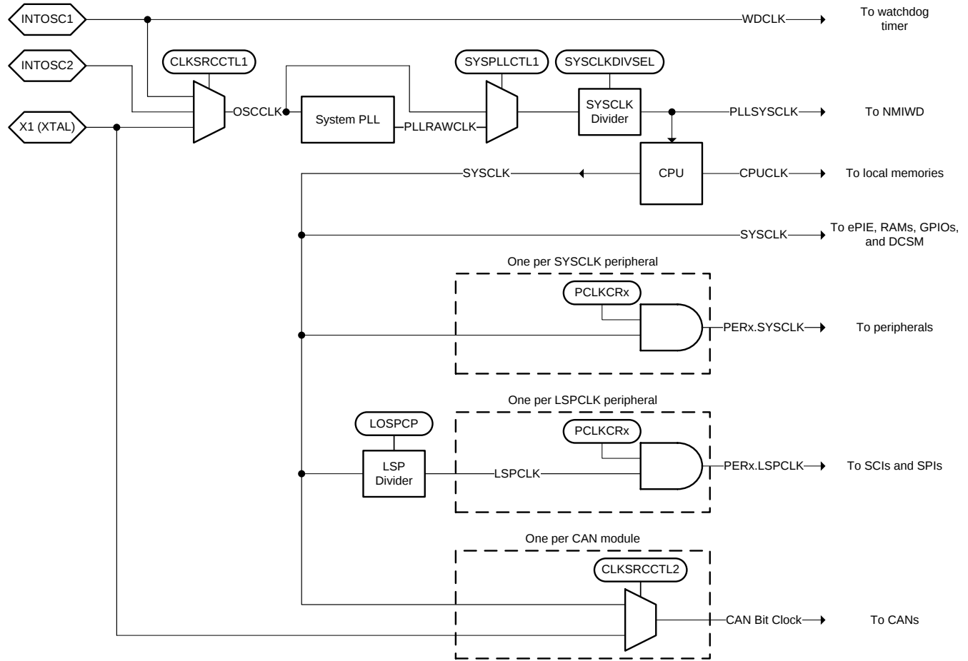
图 5-10. Clocking System
