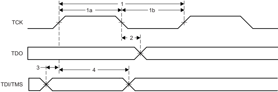
图 5-19. JTAG Timing
