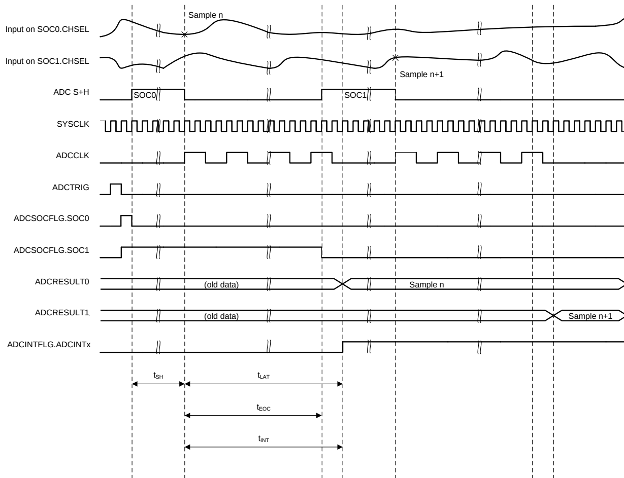
图 5-35. ADC Timings
