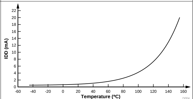
图 5-5. Halt Current Versus Temperature (°C)
