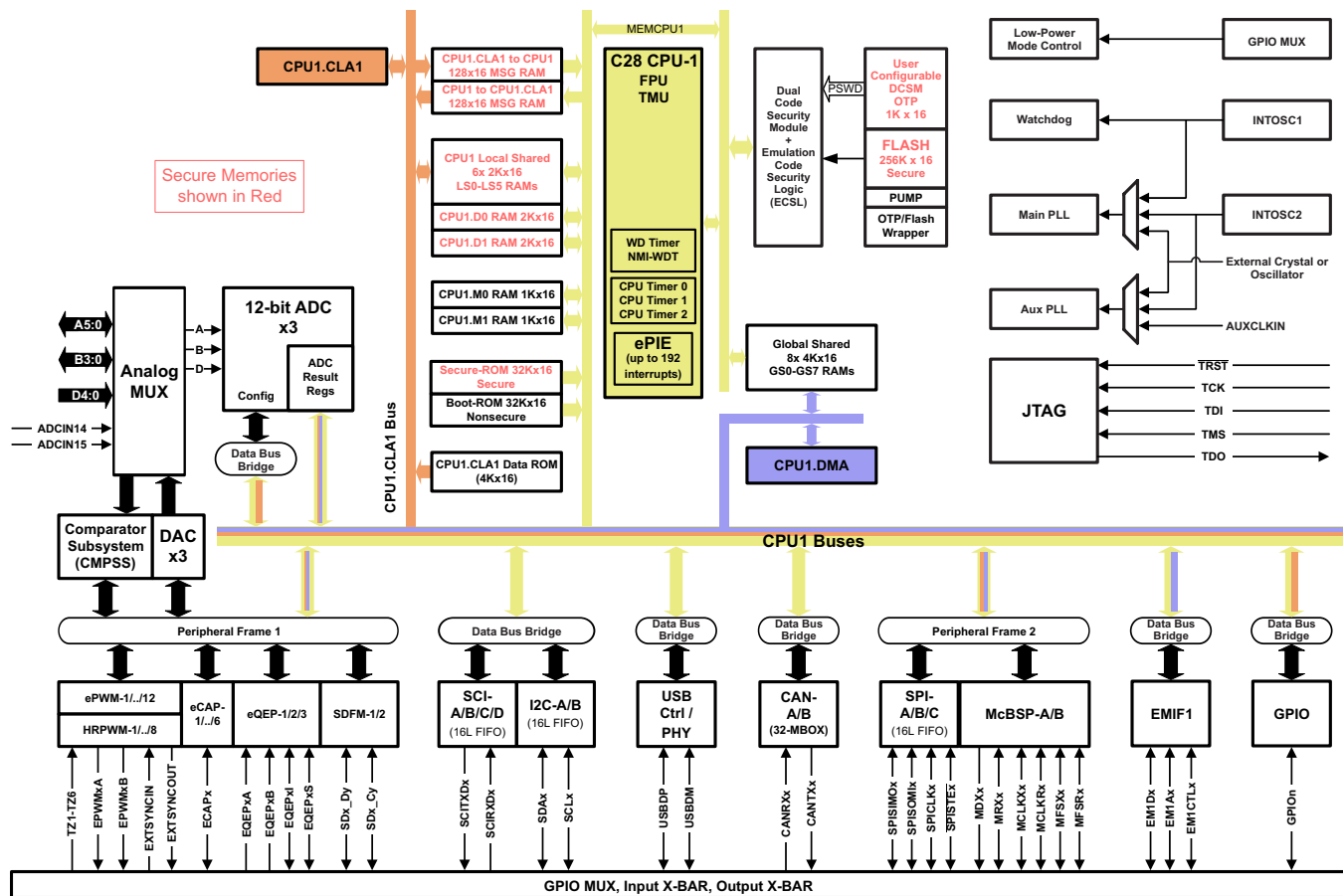
图 1-1. 功能方框图
