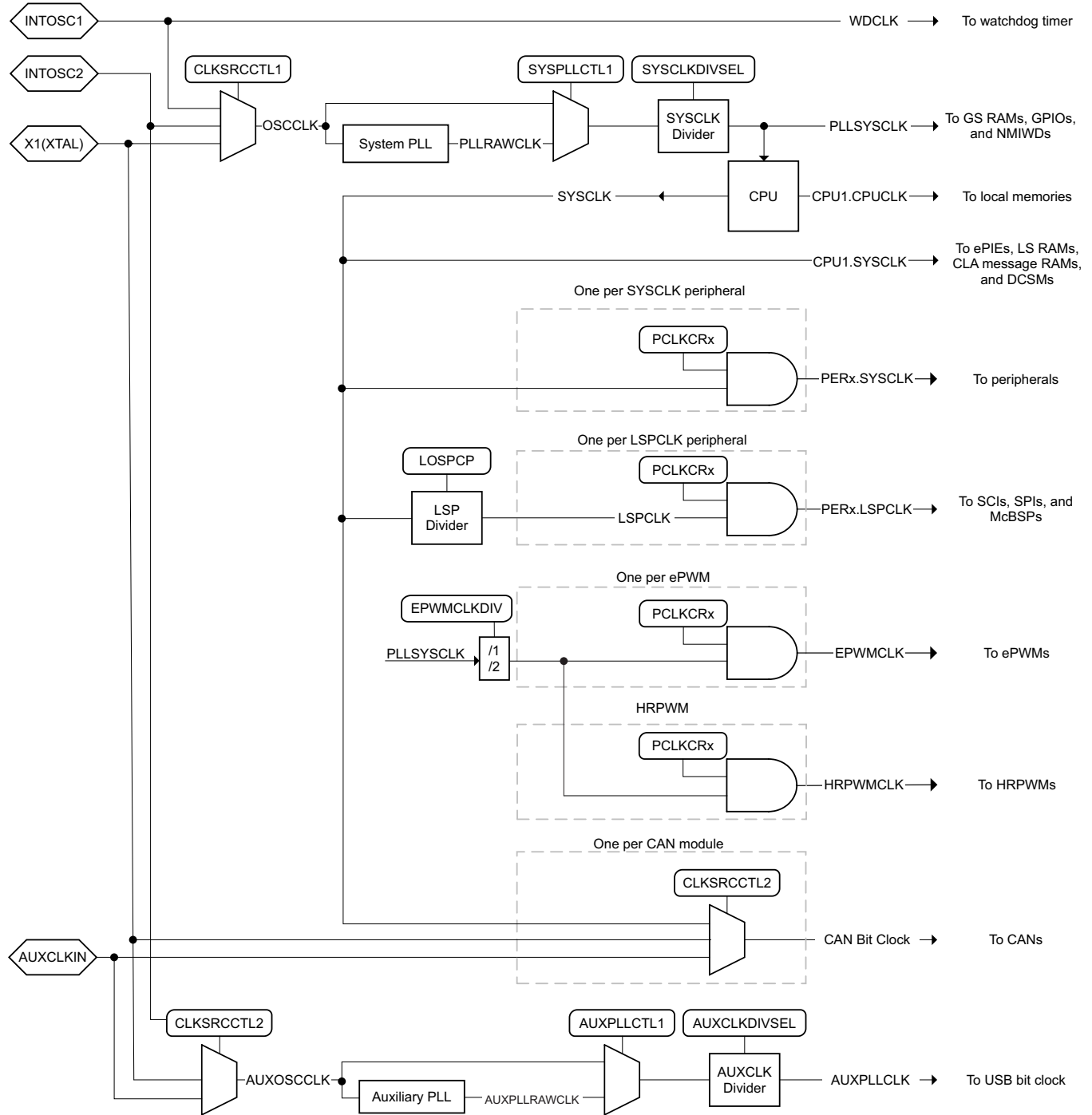
图 5-7. Clocking System
