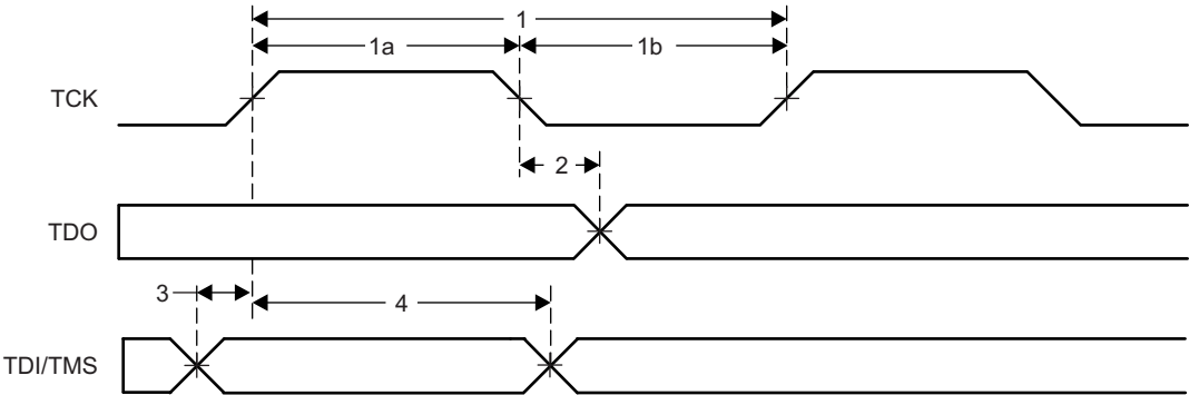
图 5-11. JTAG Timing
