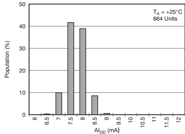
Figure 68. COMBINED AV DD AND DV DD SUPPLY CURRENT
