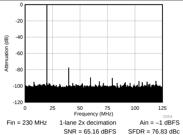
图 8. FFT 230 MHz
