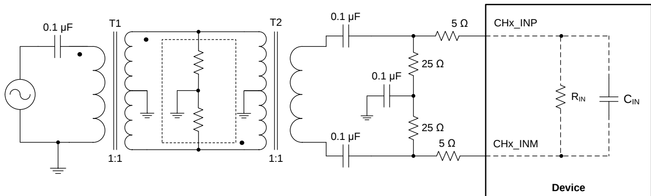
图 101. Input Drive Circuit
