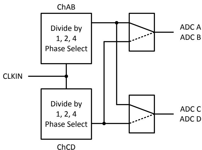
图 69. Input Clock Divider
