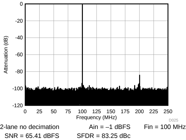
图 29. FFT 100 MHz
