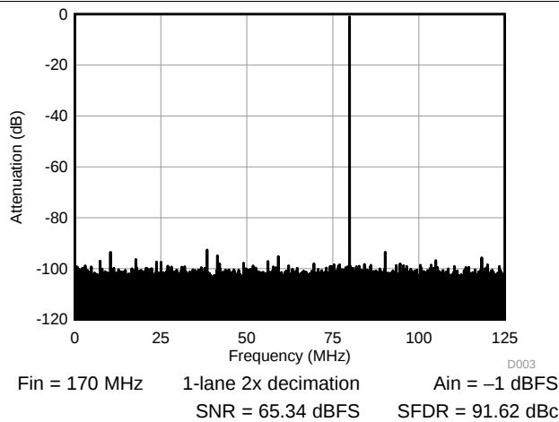
图 7. FFT 170 MHz
