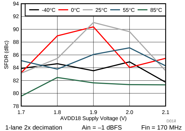
图 18. SFDR vs. AVDD18
