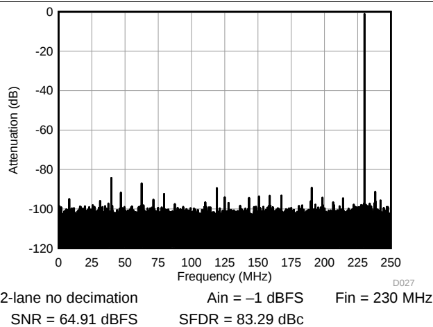
图 31. FFT 230 MHz
