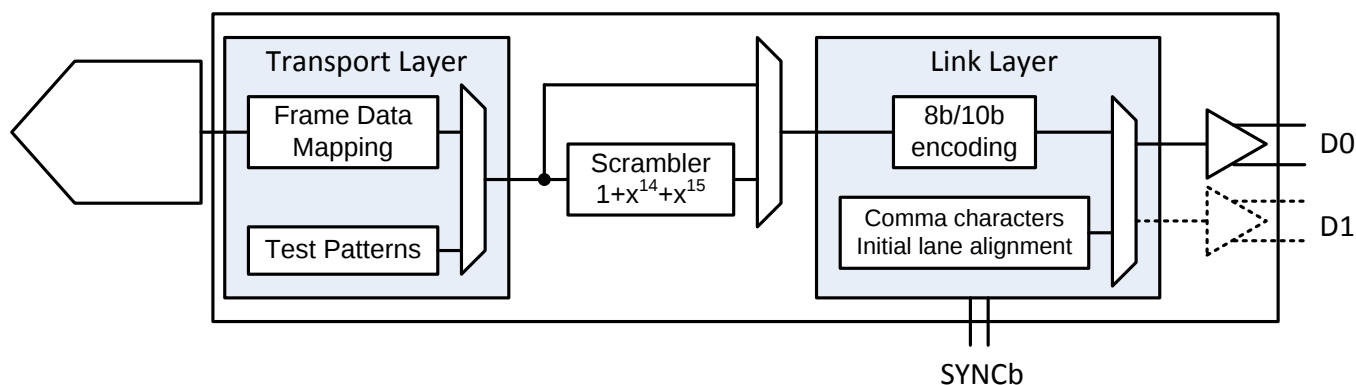
图 60. JESD204B Block
