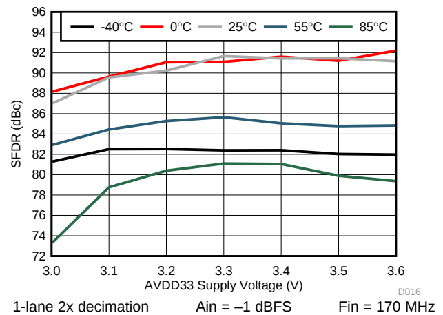
图 20. SFDR vs. AVDD33
