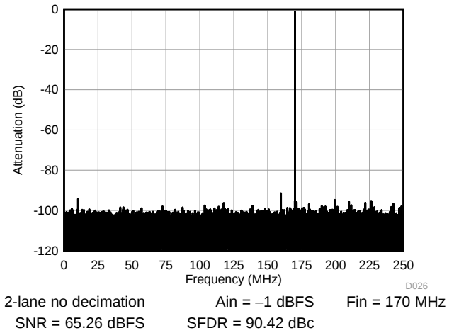
图 30. FFT 170 MHz
