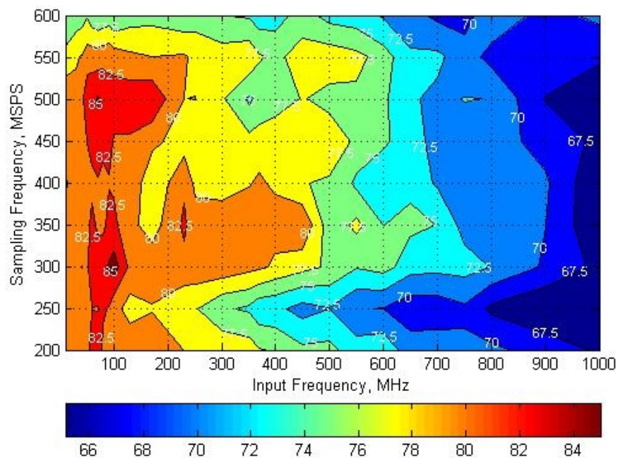
图 51. SFDR Contour Plot
