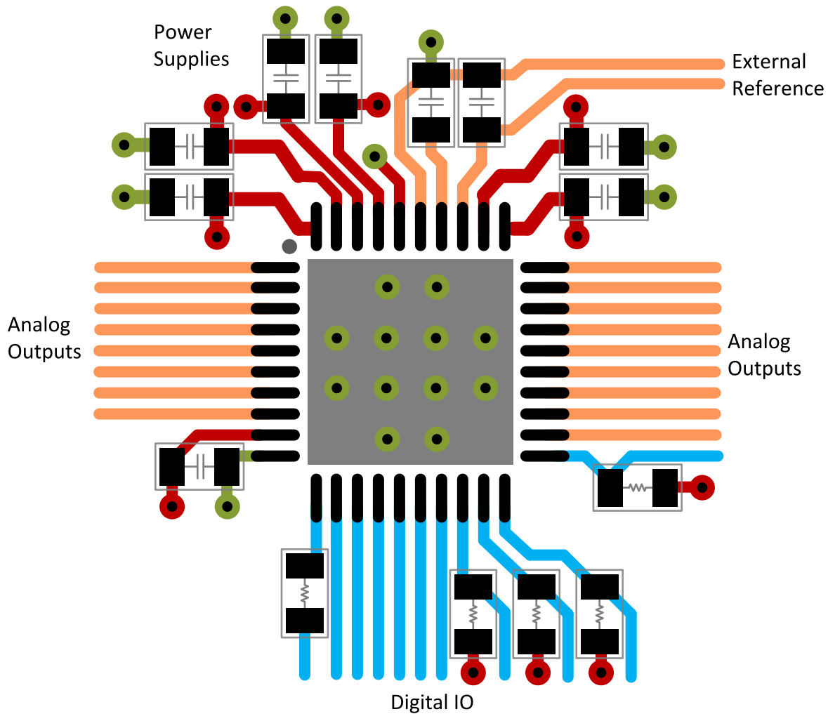
图 70. Example Layout
