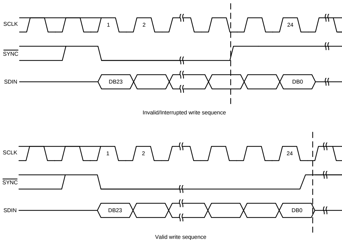
图 5. \overline{\text{SYNC}} Interrupt
