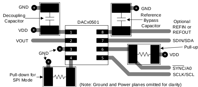
图 17. Layout Example
