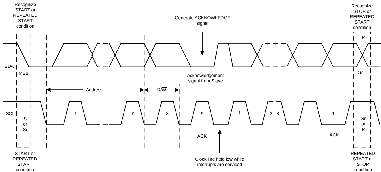
图 9. I 2 C Bus Protocol
