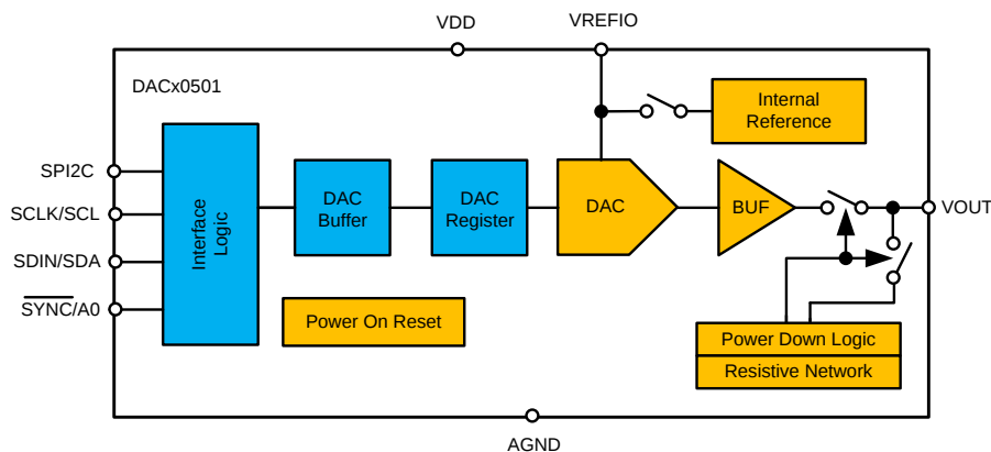
功能框图
