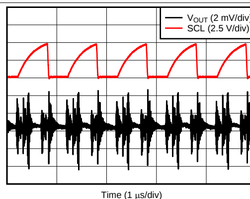
图 37. SCL = 1MHz 时的时钟馈通
