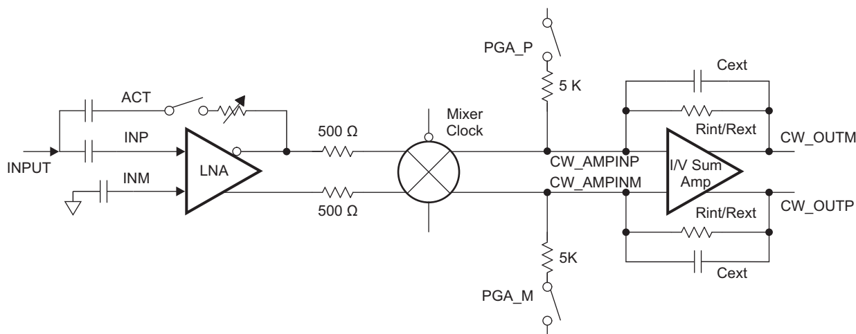
图 82. AFE5812 PGA Test Mode
