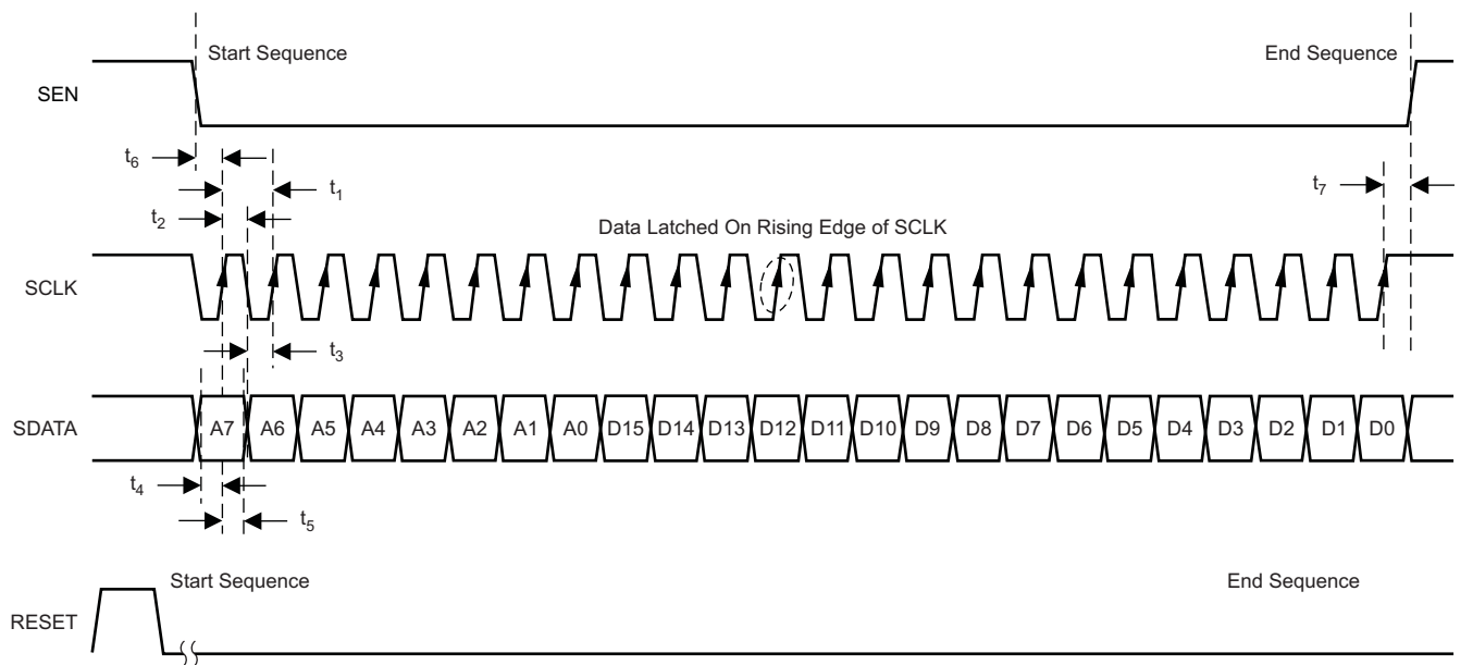
图 84. SPI Timing
