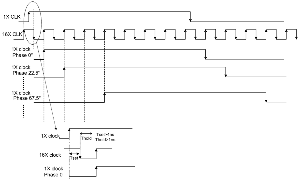
图 70. 1x 和 16x CW 时钟定时
