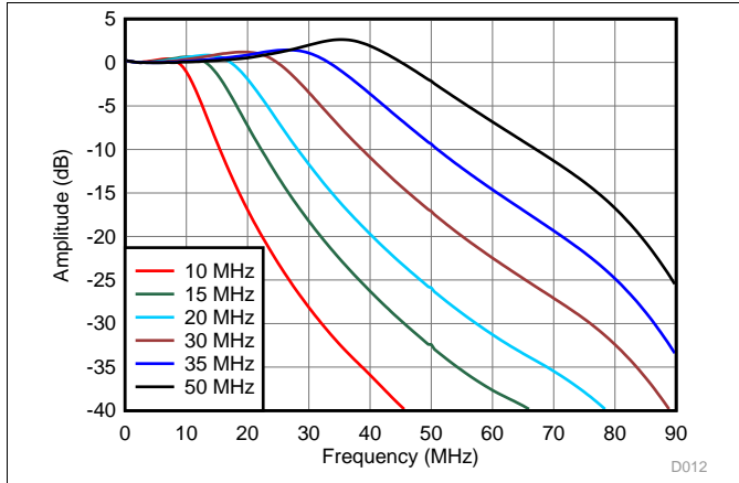
图 12. LPF Response
