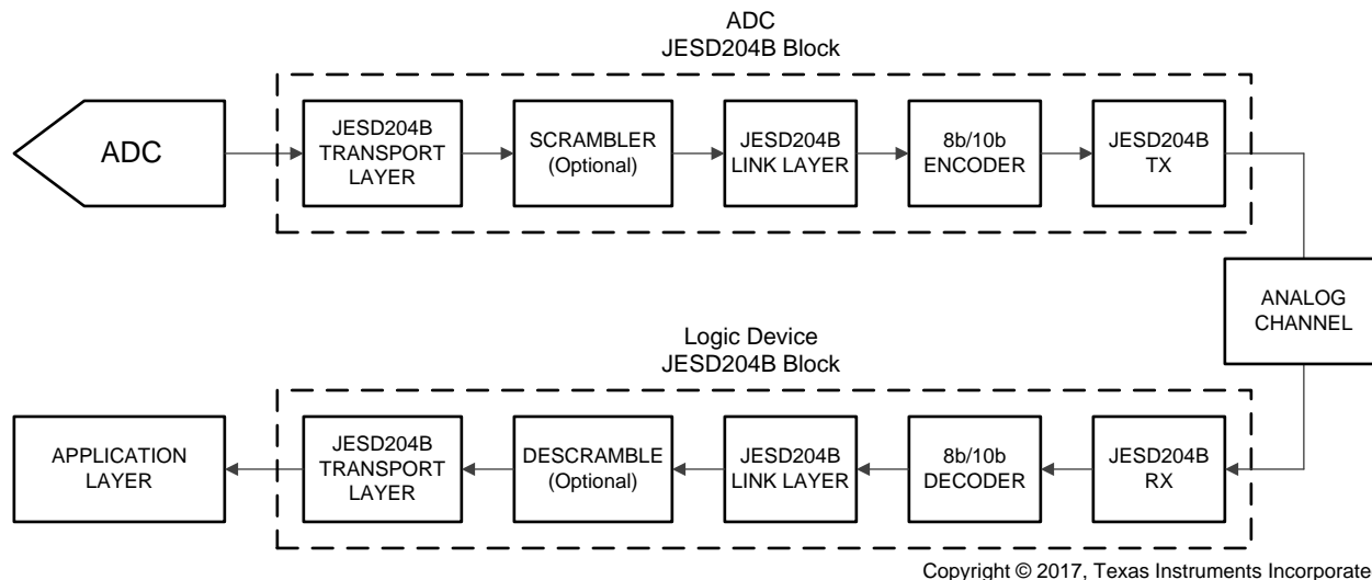
图 81. Simplified JESD204B Interface Diagram
