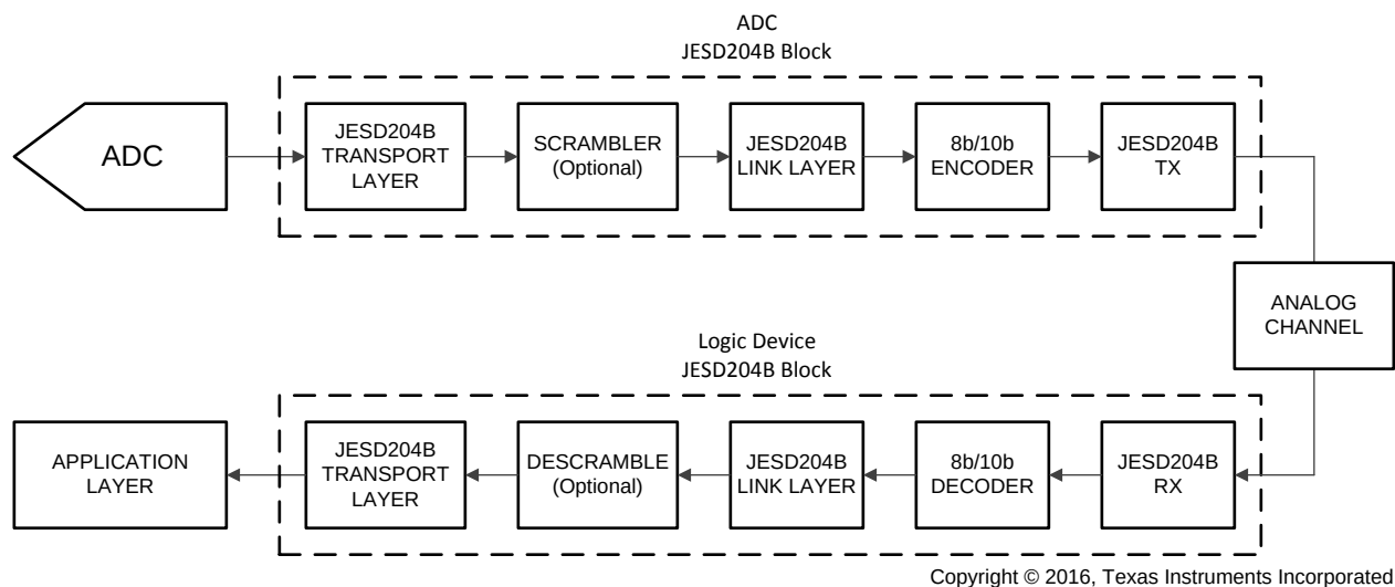
图 82. Simplified JESD204B Interface Diagram
