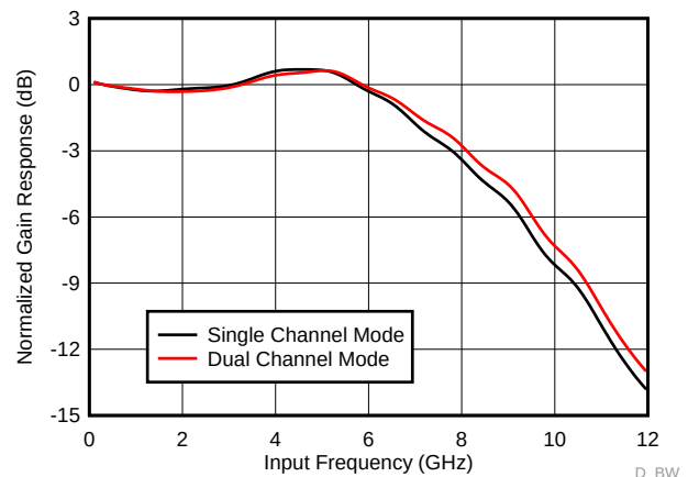
ADC12DJ3200 测量的输入带宽
