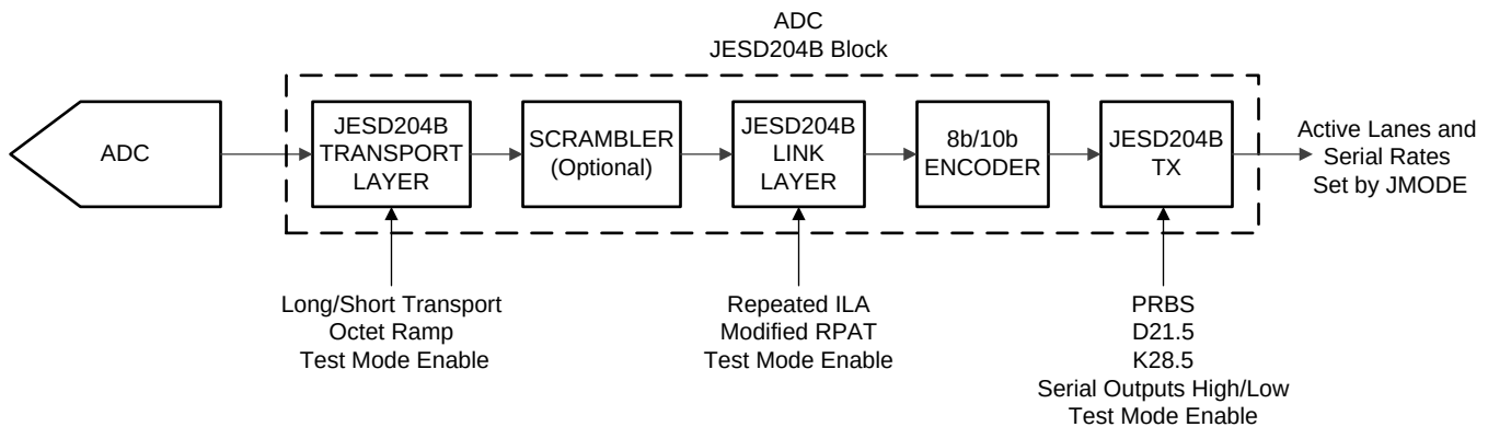
图 24. Test Mode Insertion Points
