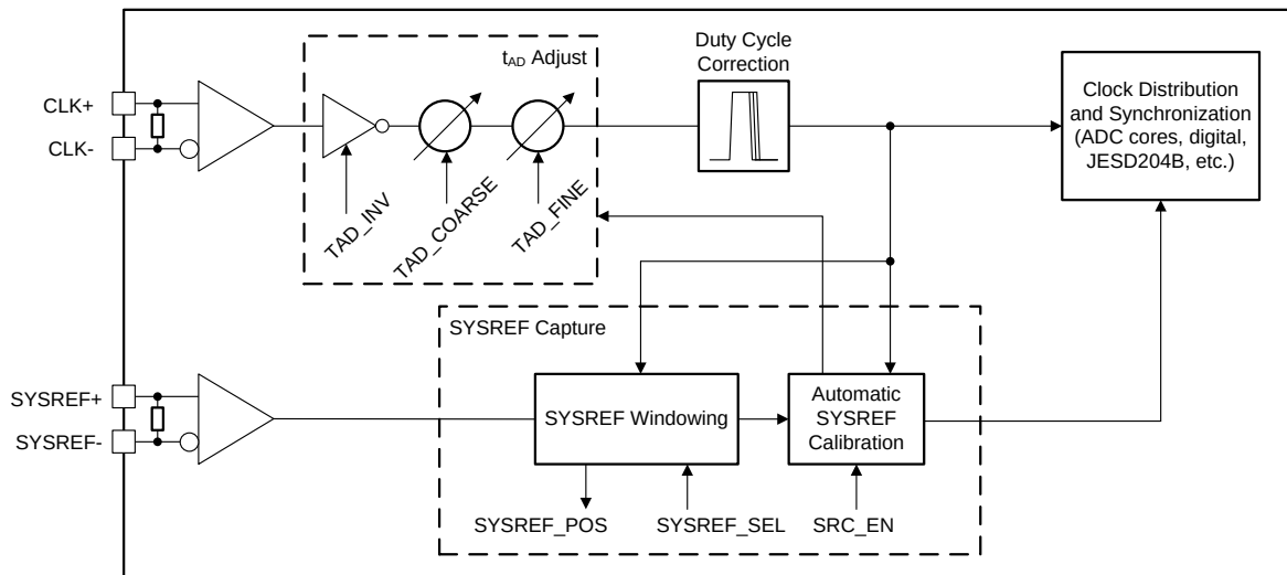
图 5. ADC12DJ3200QML-SP Clocking Subsystem
