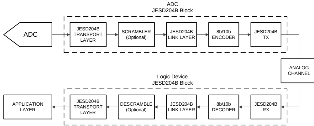
图 21. Simplified JESD204B Interface Diagram
