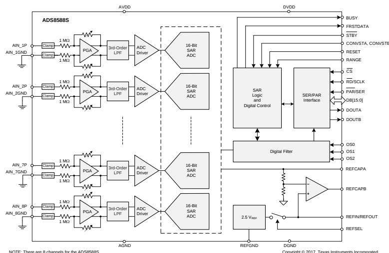
简化框图
