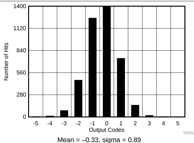
图 75. DC Histogram for OSR16
