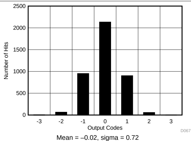
图 77. DC Histogram for OSR64
