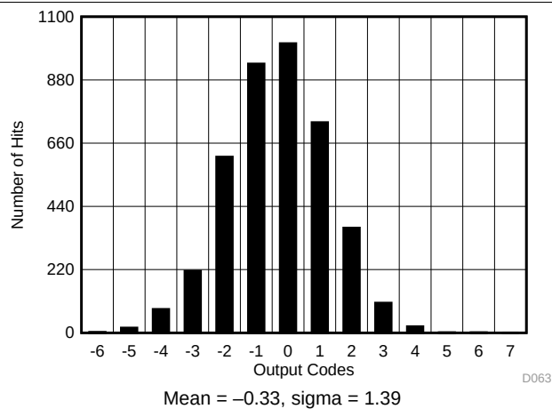
图 73. DC Histogram for OSR4
