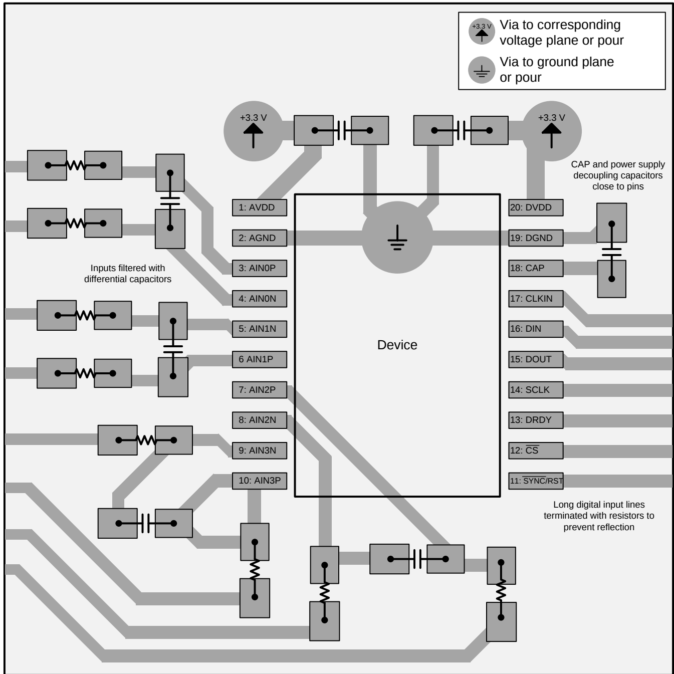
图 58. Layout Example
