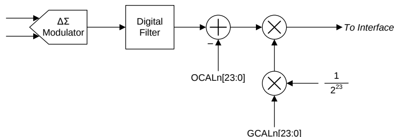
图 15. Calibration Block Diagram
