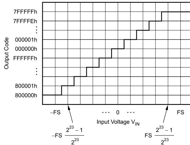
图 19. Code Transition Diagram
