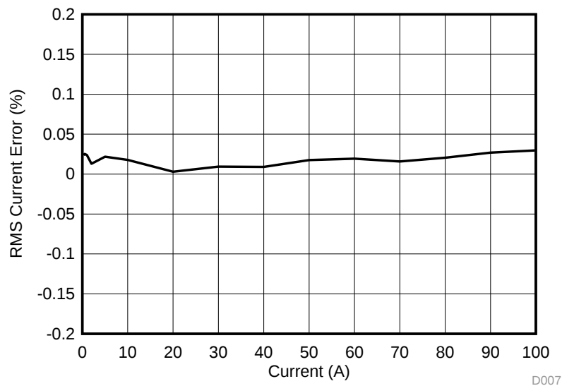
图 54. Phase B RMS Current % Error
