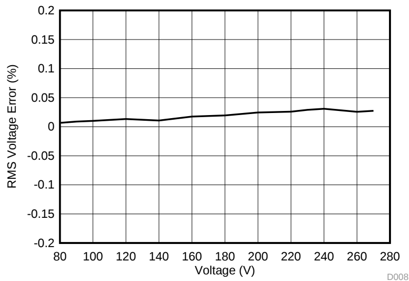
图 55. Phase A RMS Voltage % Error
