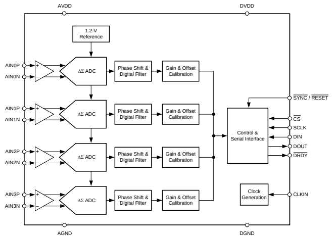
简化方框图
