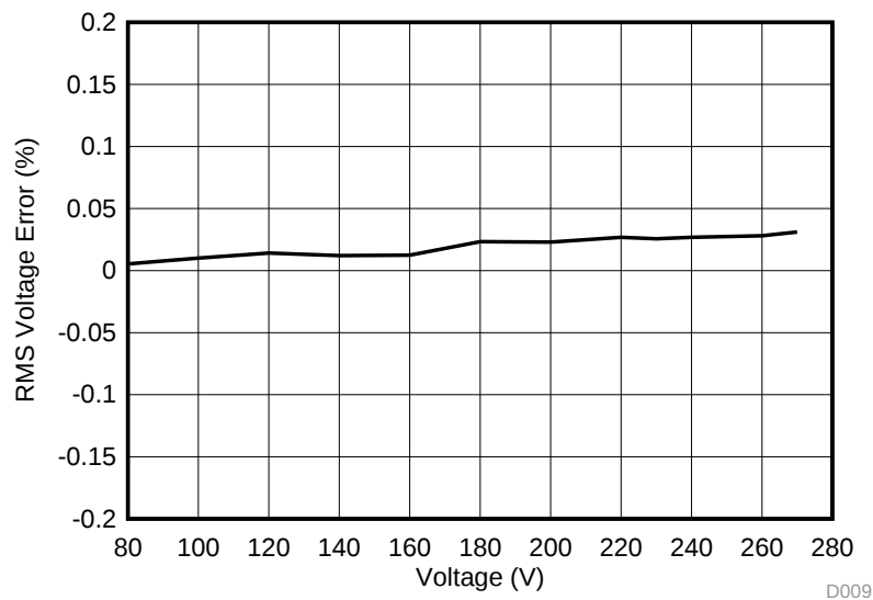
图 56. Phase B RMS Voltage % Error
