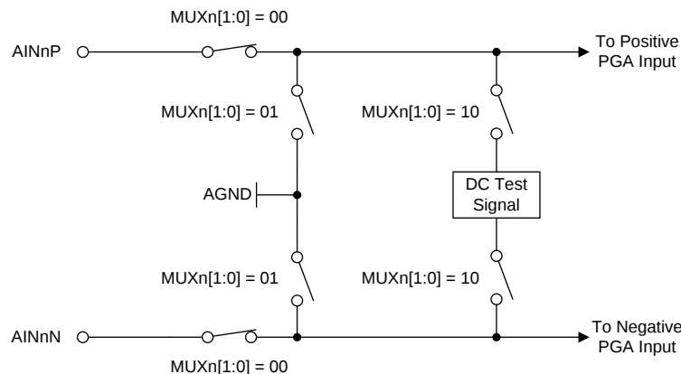
图 5. Input Multiplexer
