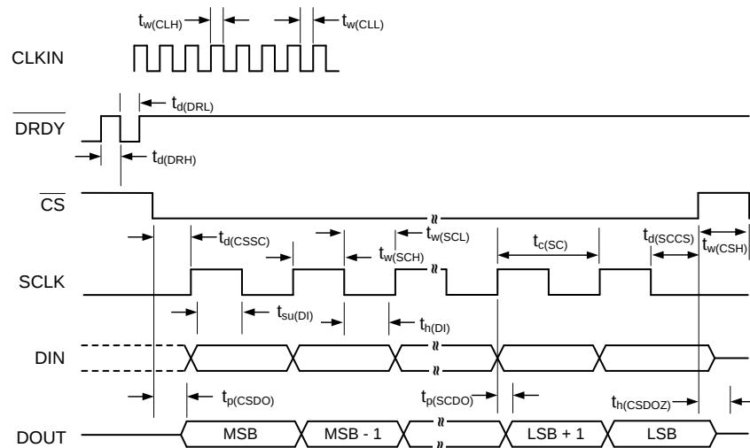
图 1. SPI Timing Diagram
