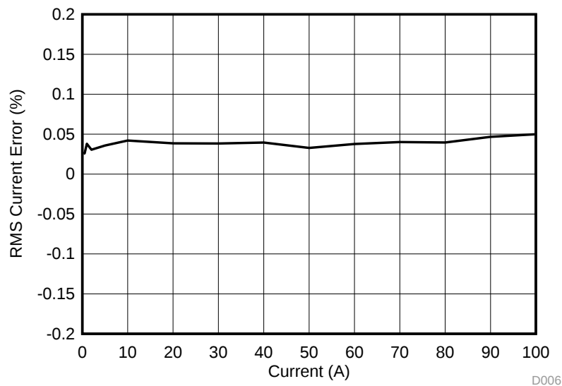
图 53. Phase A RMS Current % Error
