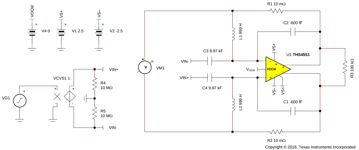
图 99. 开环增益和相位 TINA-TI™ 仿真设置
