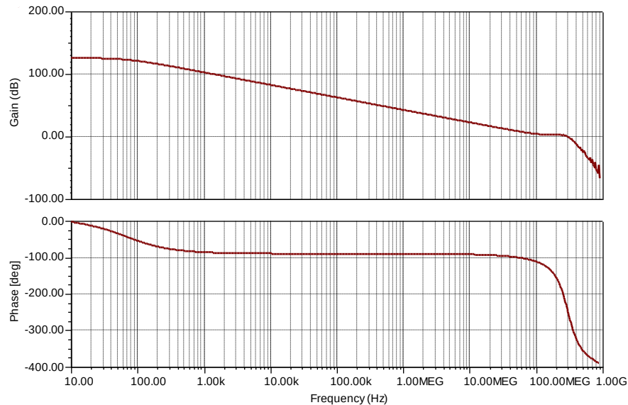
图 100. 开环增益和相位仿真结果
