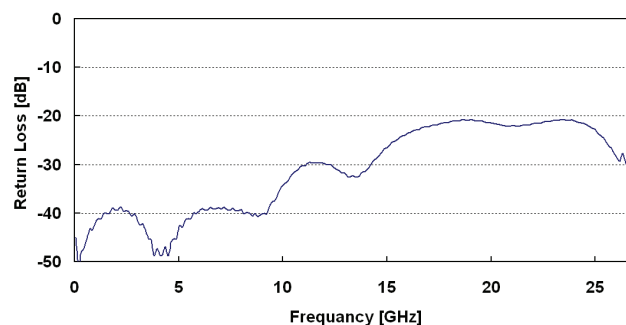
S-Parameter
