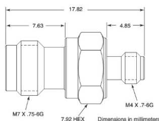
34WFVF50 outline
