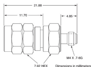
34WFV50 outline
