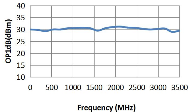
OP1dB
