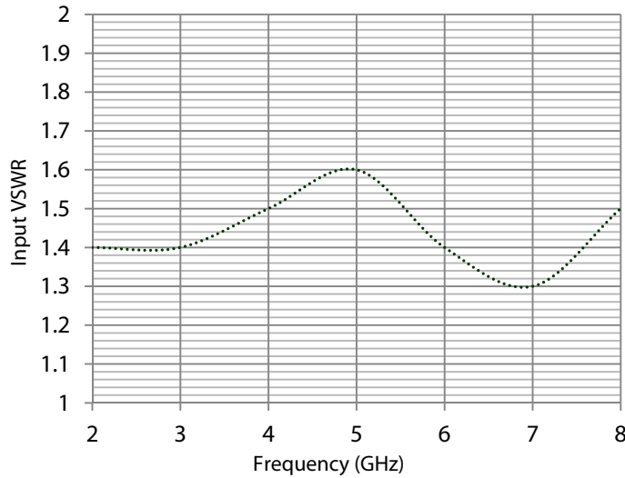
Input VSWR
