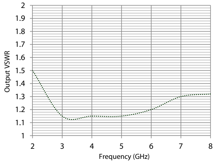
Output VSWR
