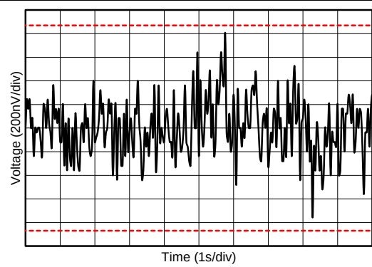
图 2. 0.1-Hz to 10-Hz Noise
