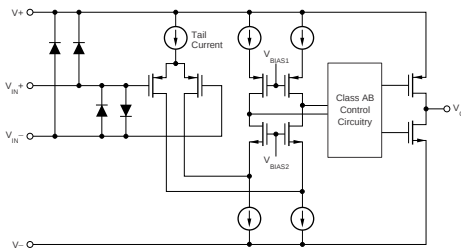
简化内部原理图
