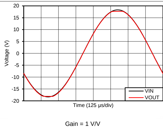
图 30. No Phase Reversal
