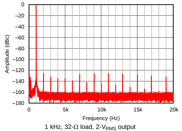
图 45. Output Spectrum
