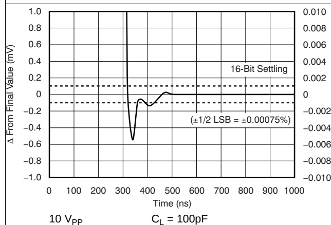
图 31. 大信号正极性建立时间
