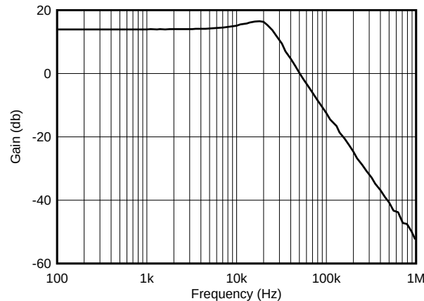
图 50. OPAx211 二阶 25kHz 切比雪夫低通滤波器
