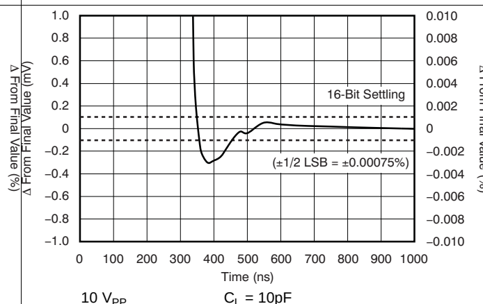
图 32. 大信号正极性建立时间
