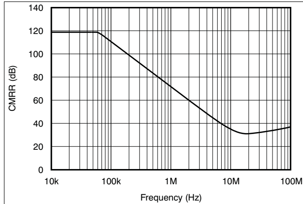
图 7. 共模抑制比与频率间的关系
