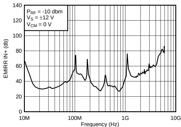
图 46. OPA211 EMIRR
