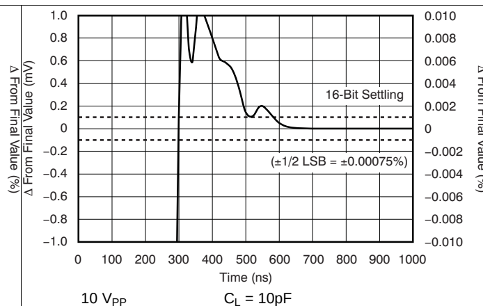
图 32. 大信号正极性建立时间
