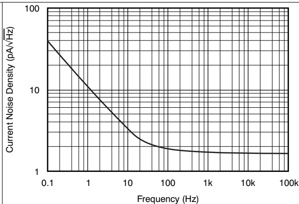
图 2. 输入电流噪声密度与频率间的关系
