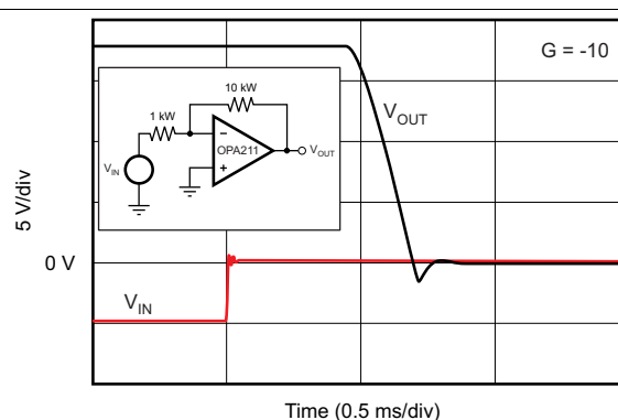
图 34. 大信号负极性建立时间
