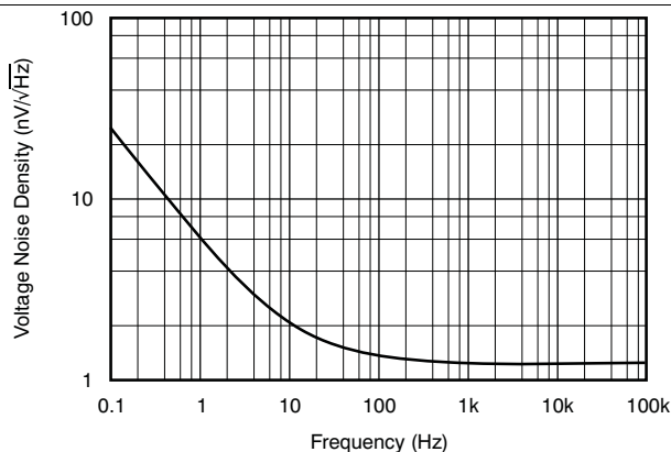
图 1. 输入电压噪声密度与频率间的关系
