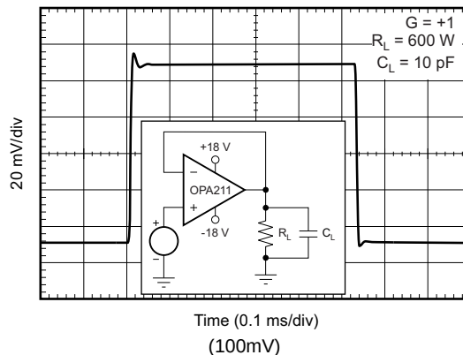
图 26. 小信号阶跃响应
