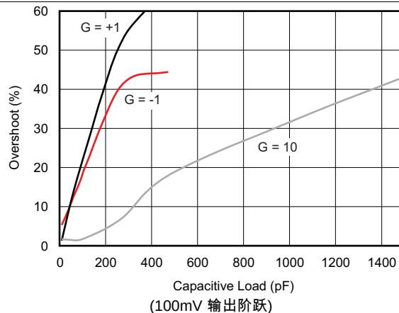
图 28. 小信号过冲与容性负载间的关系
