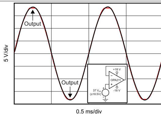
图 38. 无相位反转
