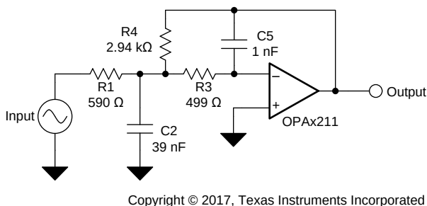
图 49. OPAx211 简化原理图
