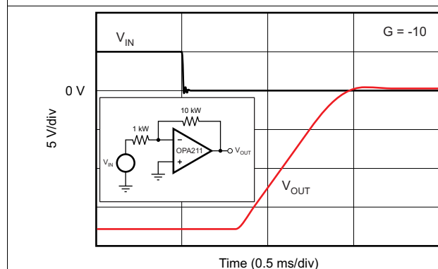
图 33. 大信号负极性建立时间
