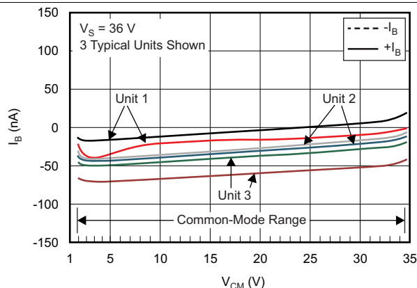
图 19. 输入偏置电流与共模电压间的关系
