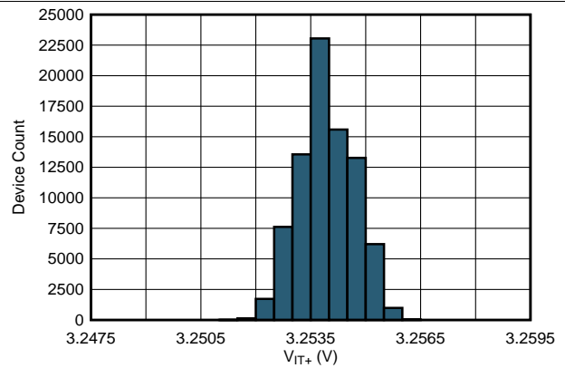
TLV4021S5
