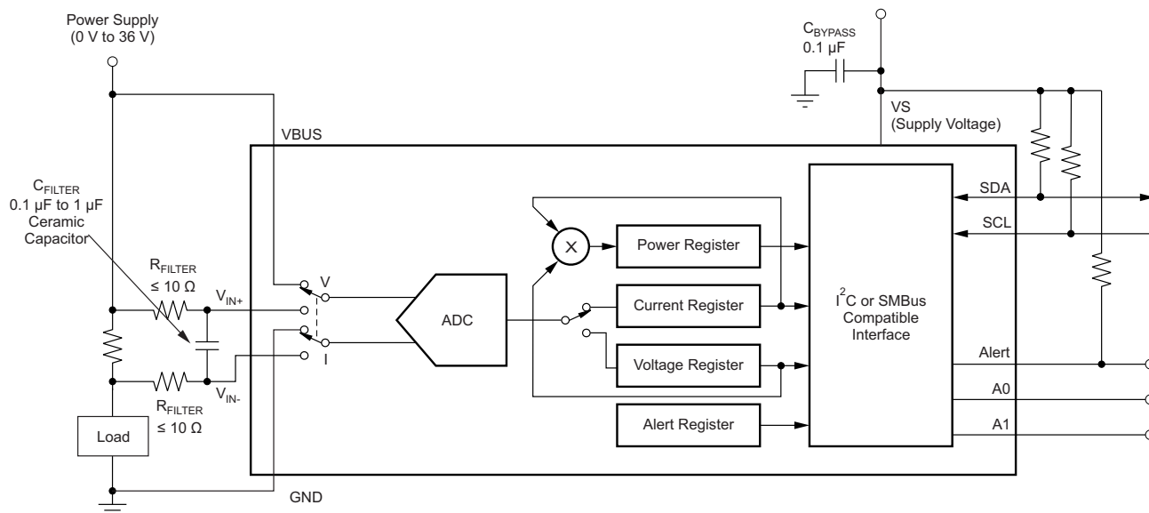
图 21. Input Filtering
